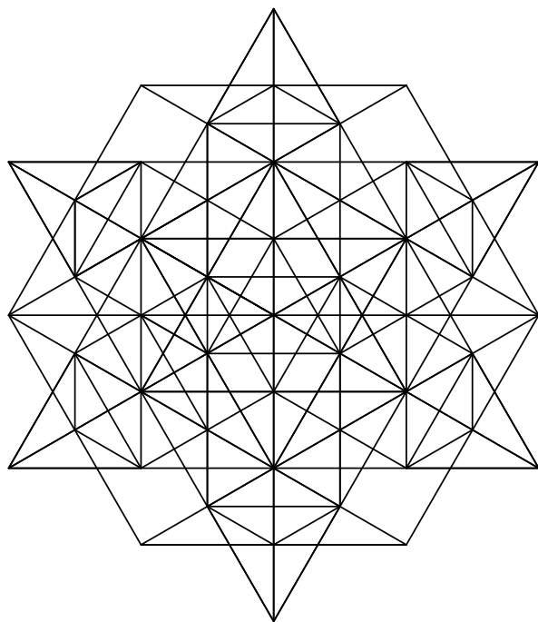
Izotropna vektorska matrica
